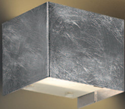
2765.01FA 1 luce - Foglia argento L. 11,5 x 9 S. 8 cm. G9 #1x40W oppure 1 LED 10W - 300MA - Natural
