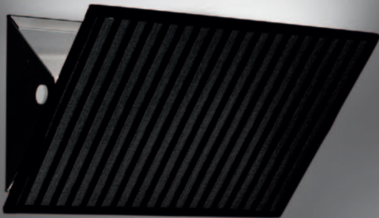
2776.01 1 luce Schermo orientabile L. 14 x 19 S. 7 cm. R7s 118mm.#1x100W
