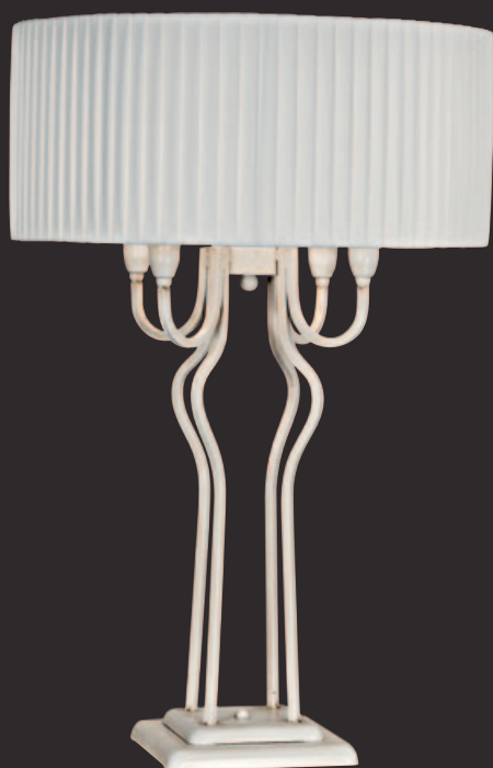
2755.05AA 4+1 luci - Avorio anticato Ø 50 H. 75 cm. E14#5x40W
